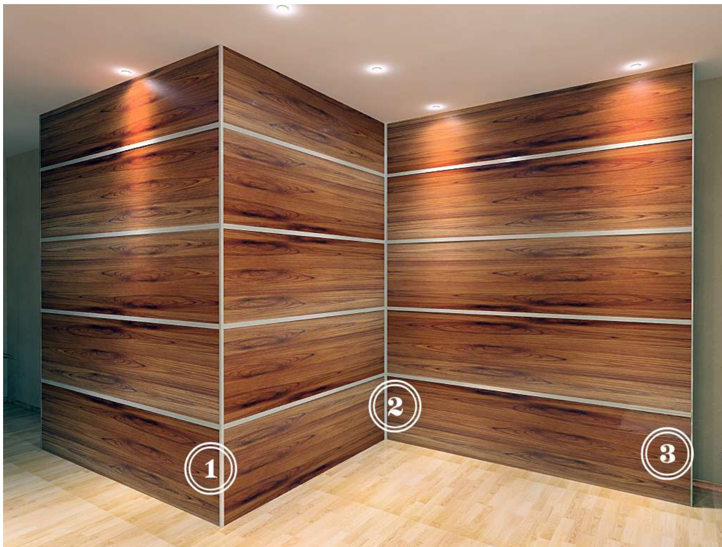
Система стеновых панелей с открытым профилем (Омега/Пи)
